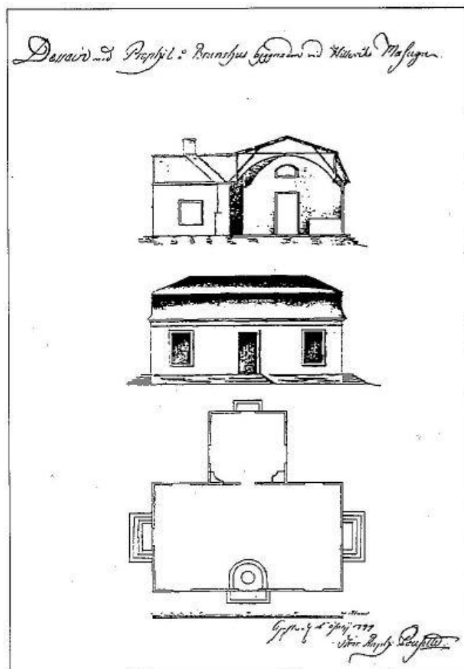
Plan och sektioner till brunnshusbyggnaden vid Hilleviks hälsokälla. Ritning gjord 1799 av J.P. Pousette. EFTER FOTO I NORDISKA MUSEET. HERRGÅRDSINVENTERINGEN. Originalen i karmin, krongult och laving.
